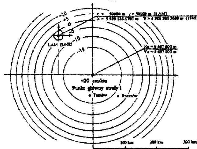
Rys. 4. Położenie układu lokalnego miasta Łodzi (ŁAM) na tle izolini zniekształceń liniowych w strefie I układu 1965, obrazujące zmienność skali w transformacji xy_{LOK} \Leftrightarrow xy_{65}
